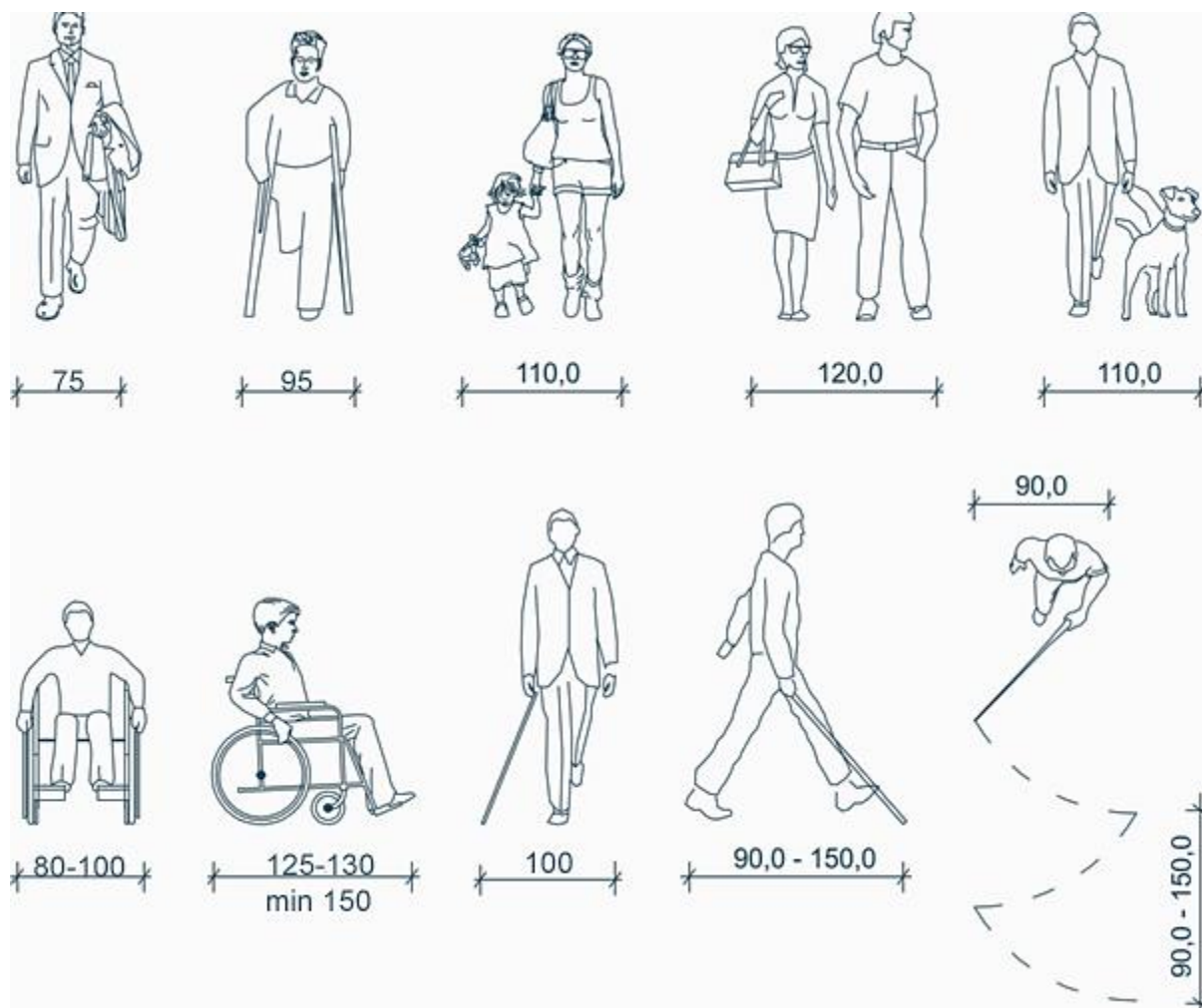
Rys. 03. Minimalne wymiary skrajni ruchu poszczególnych użytkowników [wymiaru podane w cm]
