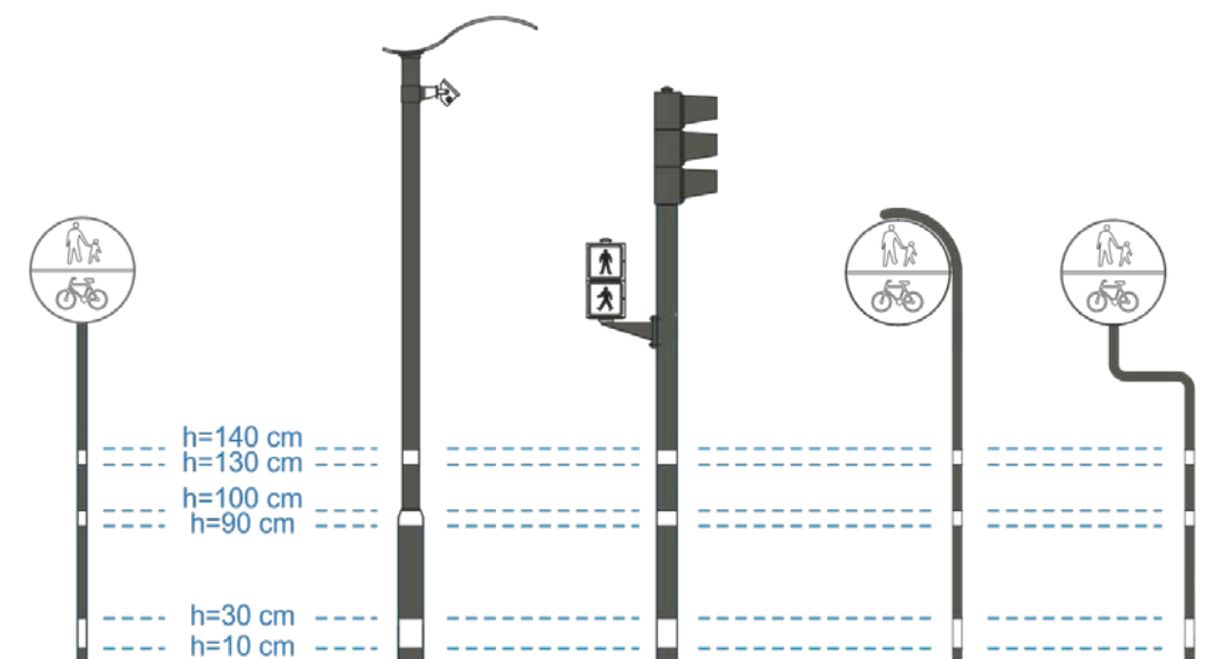
Rys. 09. Schemat oznaczeń kontrastowych pionowych elementów w przestrzeni oraz przykłady montażu znaków drogowych na wygiętych sztycach
