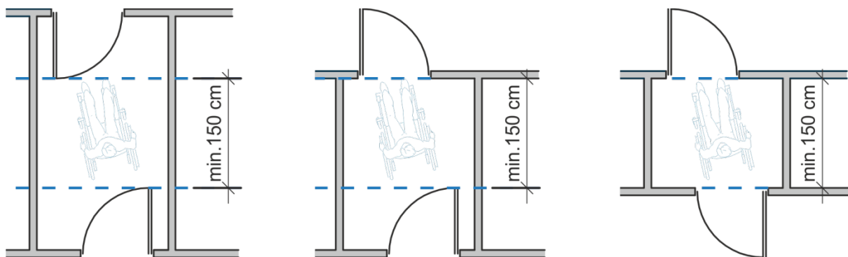
Rys. 38. Minimalne wymiary korytarzy i przedsionków w zależności od kierunku otwierania drzwi
