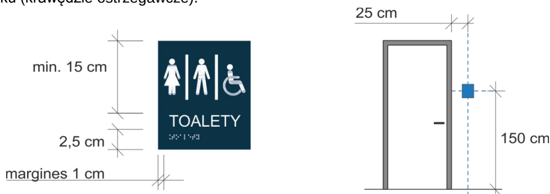
Rys. 58. Wytyczne dla oznaczeń ściennych: wymiary oraz sposób montażu oznaczeń
