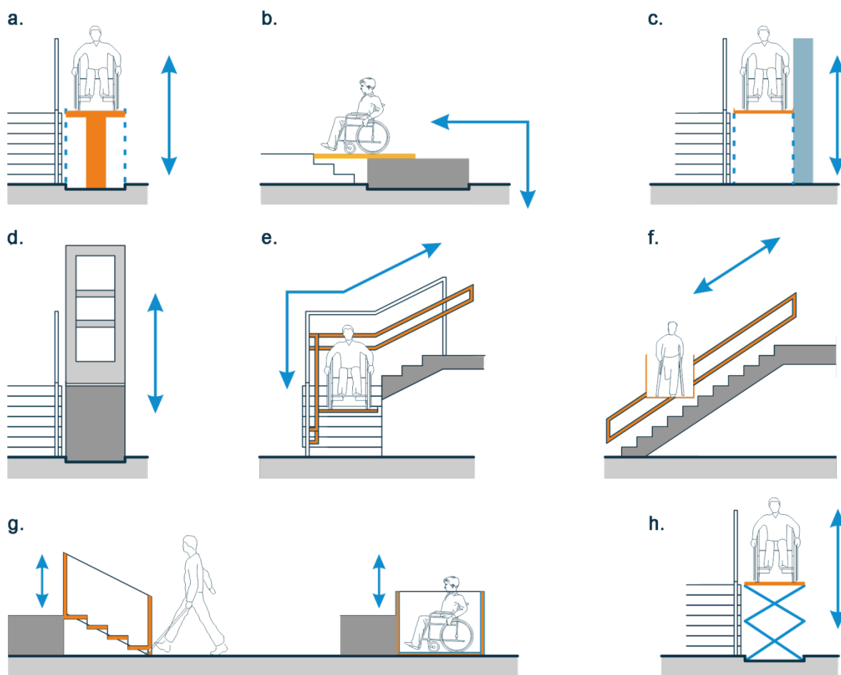
Rys. 33. Przykłady podnośników i platform
