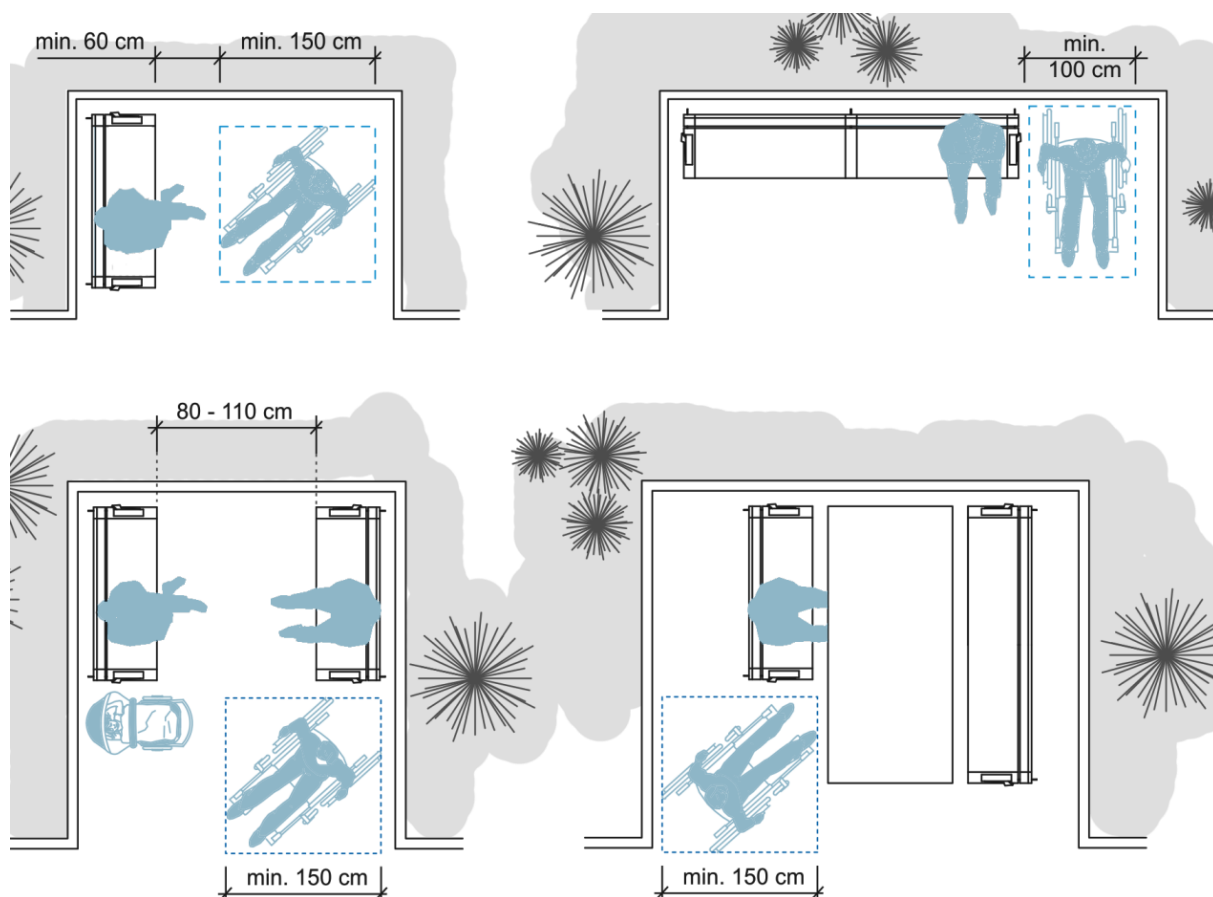
Rys. 45. Przykładowe rozwiązania miejsc odpoczynku w obrębie parków i skwerów
