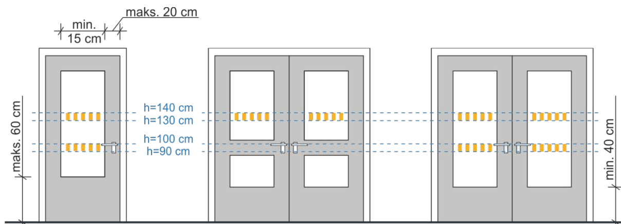
Rys. 36. Przykładowe oznaczenie elementów szklanych i lokalizacja informacji graficznej
