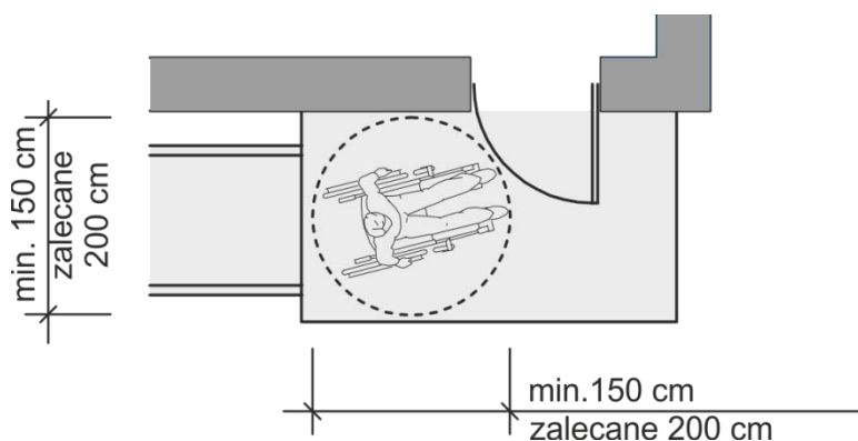
Rys. 25. Powierzchnia manewrowa na spocniku pochylni
