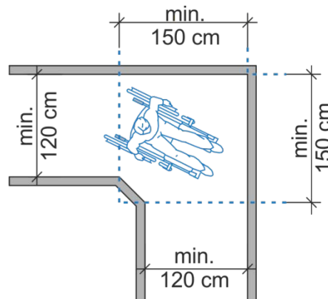
Rys. 39. Przykład rozwiązania zmiany kierunku korytarza ze sfazowanym narożnikiem
