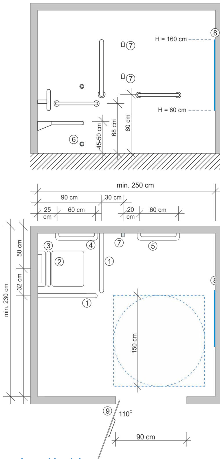
Rys. 44. Wyposażenie przebieralni
