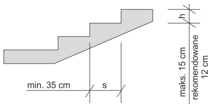
Rys. 22. Podstawowe wytyczne dla stopni schodów zewnętrznych
