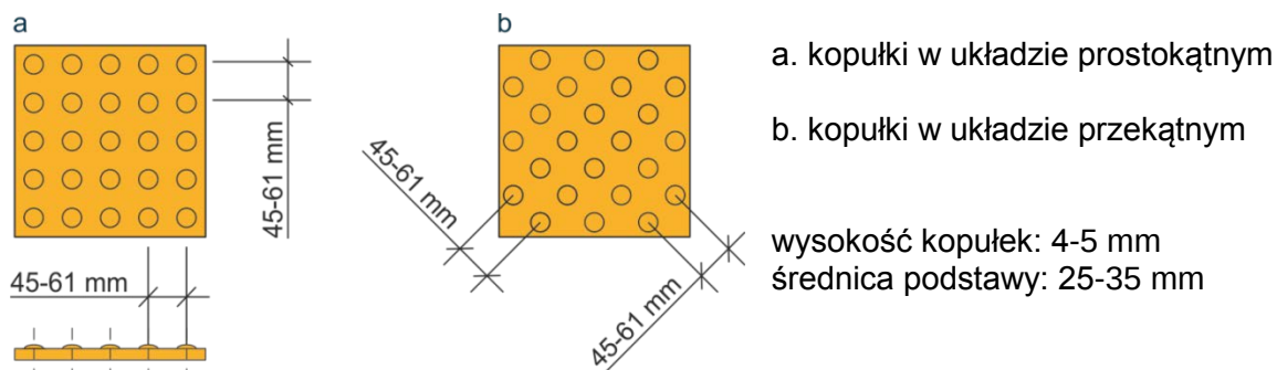
Rys. 06. Faktura ostrzegawcza – kopułkowa – opracowanie własne na podstawie Normy ISO 21542:2011
