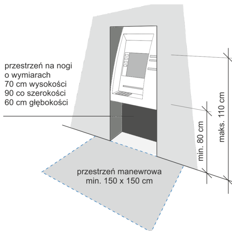
Rys. 53. Podstawowe wymiary dla automatów i urządzeń w przestrzeni miejskiej
