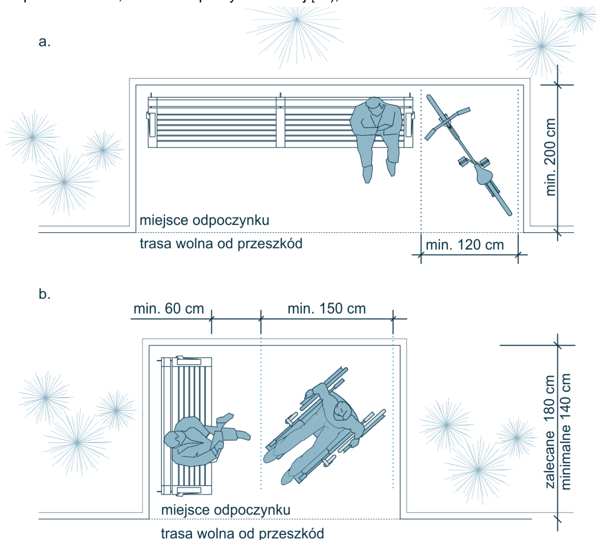
Rys.52. Przykłady aranżacji miejsc odpoczynku z miejscem dla roweru (a) i wózka (b) nieuwzględniające lokalizacji kosza na śmieci
