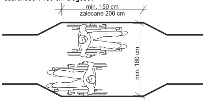
Rys. 12. Schemat rozwiązania poszerzenia ciągu pieszego
