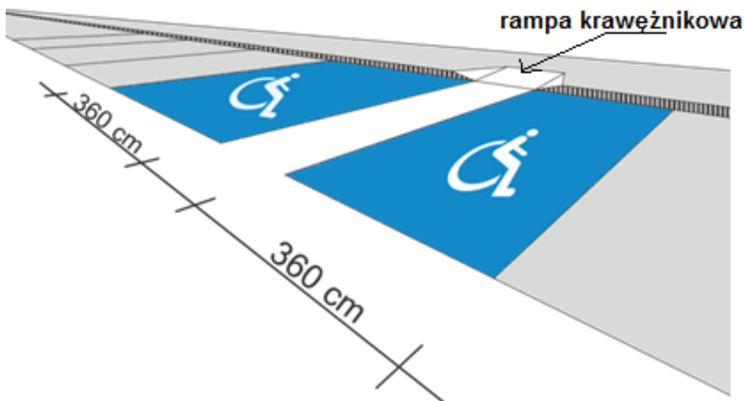
Rys. 16. Przykład zapewnienia dojścia / dojazdu do chodnika
