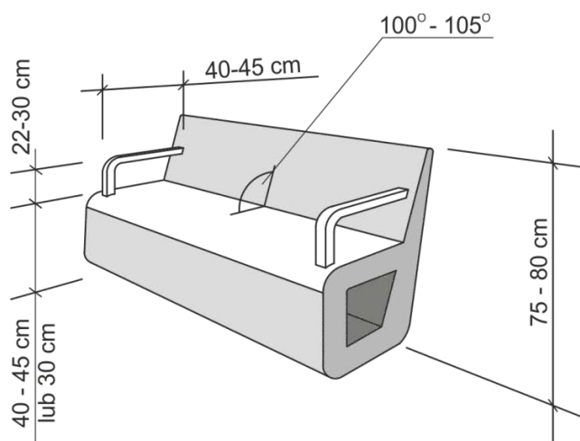
Rys. 50. Przykład ławki z podłokietnikami (z lewej)
