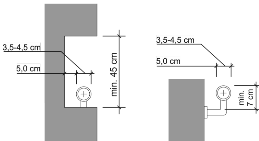
Rys. 28. Podstawowe wymagania wymiarowe dla pochwytów poręczy
