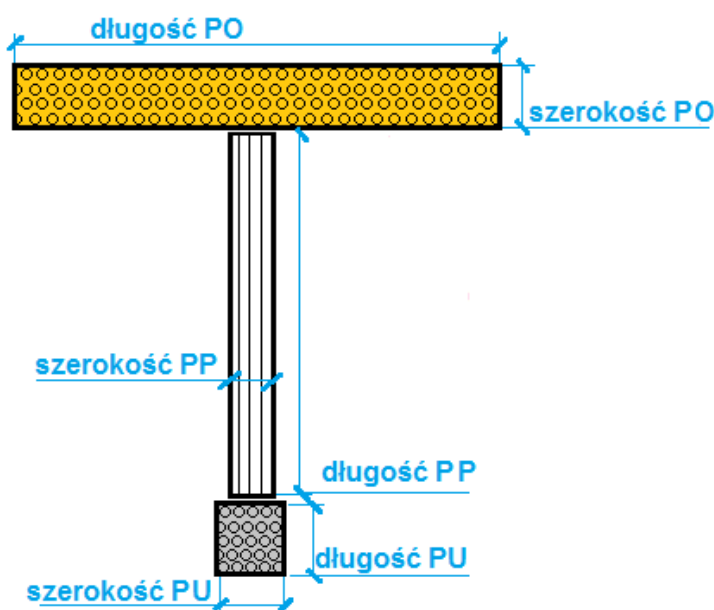
Rys. 04. Schemat systemu prowadzenia z oznaczeniem faktury ostrzegawczej PO pas ostrzegawczy, PU pola uwagi, faktury prowadzącej PP pas prowadzący - opracowanie własne
