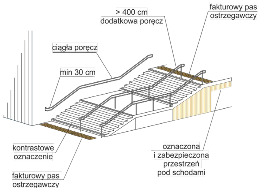
Rys. 24. Oznaczenie schodów zewnętrznych
