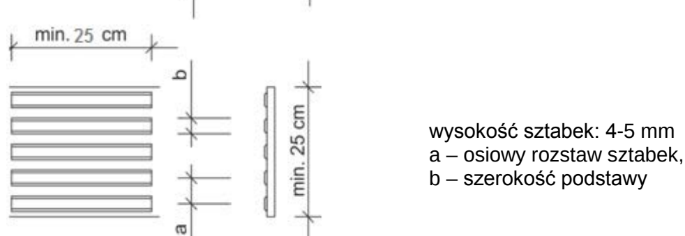
Rys. 07. Faktura prowadząca – sztabki – opracowanie własne na podstawie Normy ISO 21542:2011
