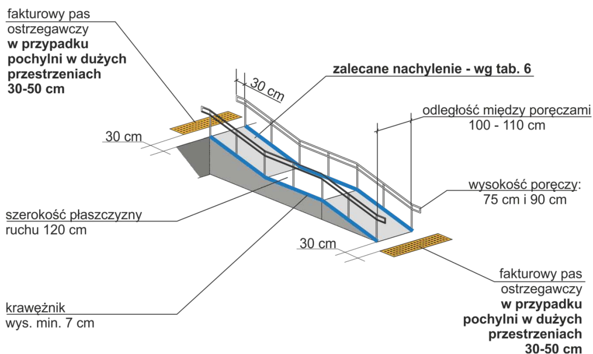
Rys. 26. Wymiary i oznaczenie pochylni
