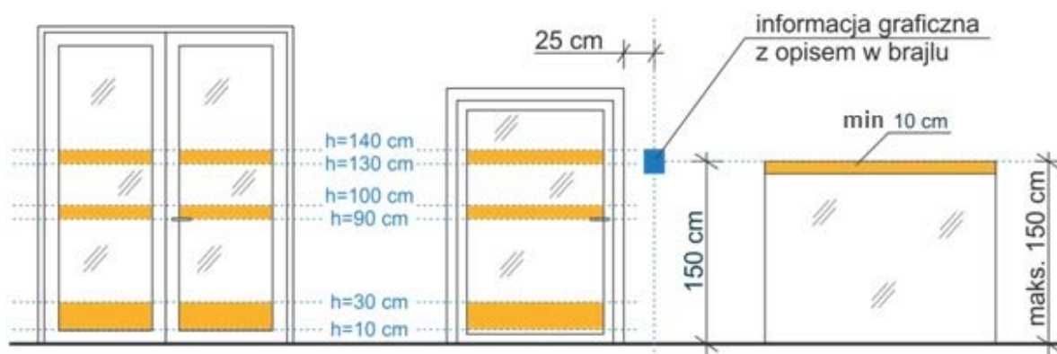
Rys. 35. Przykładowe oznaczenie elementów szklanych i lokalizacja informacji graficznej z opisem w brajlu
