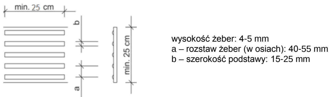
Rys. 08. Faktura prowadząca – żebra pojedyncze – opracowanie własne na podstawie Normy ISO 21542:2011
