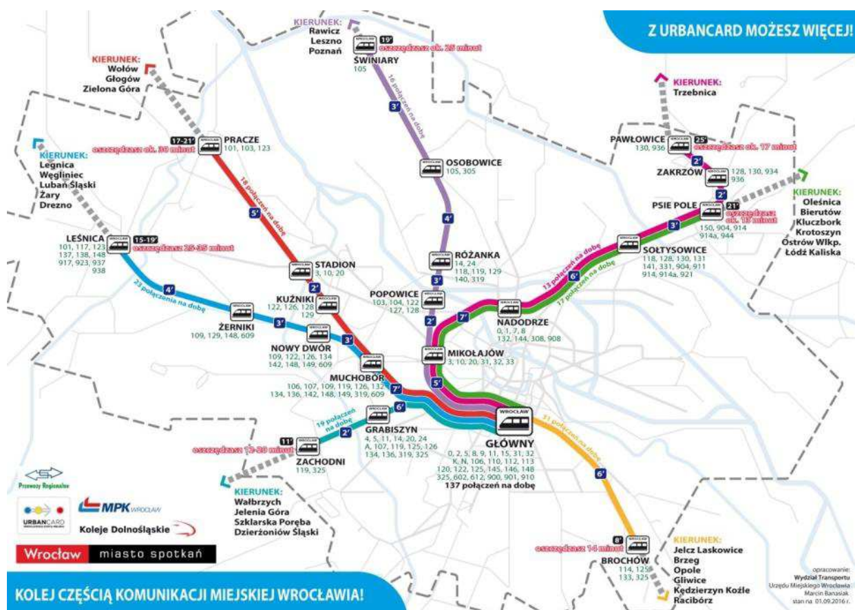
Rysunek 4: Schemat układu linii aglomeracyjnych Kolei Dolnośląskich i Kolei Regionalnych obsługiwanych we współpracy z Miastem Wrocław
