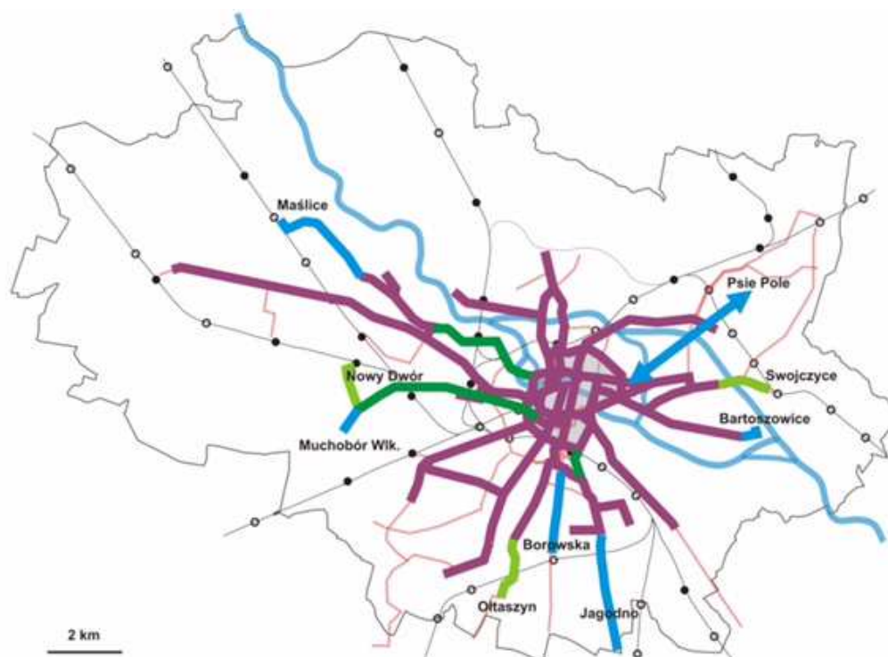
Rysunek 5: Schemat kierunków rozwoju sieci tramwajowej do dalszych analiz według WPT.
