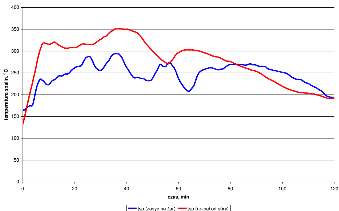
Rys. 6. Temperatura spalin mierzona na wylocie z kotła (w czopuchu) podczas spalania drewna w kotle komorowym
